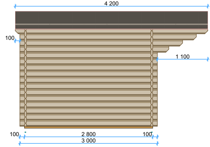
Right Elevation
